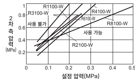
●배압에 대한 설정 압력 범위
