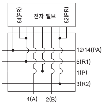
밸브 블록 단품 회로도
