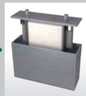
⑰ 셀 케이스 삽입 권회체를 셀 케이스에 삽입합니다.
