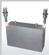
⑱ 셀 덮개 용접 셀 케이스와 덮개를 레이저로 용접합니다.
