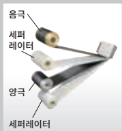
⑭ 권회 양극과 음극 사이에 세퍼레이터를 끼워 넣고 감습니다.
