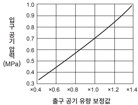
입구 압력-출구 유량 보정 곡선
