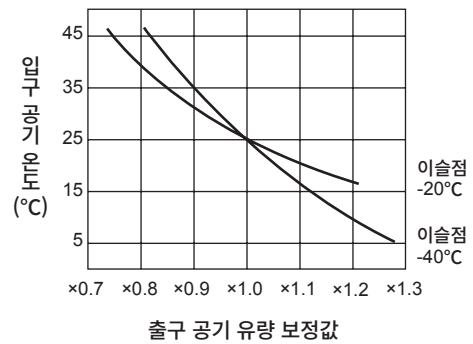
입구 온도-출구 유량 보정 곡선
